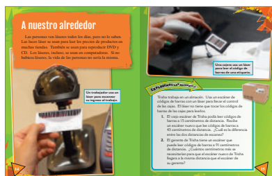
Láseres
